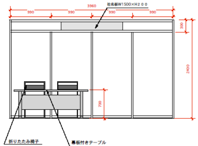
立面図
