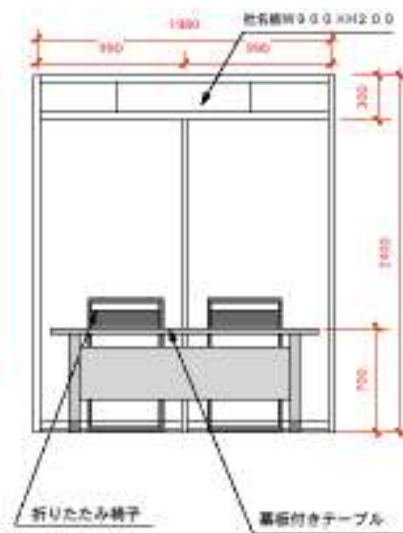
立面図
